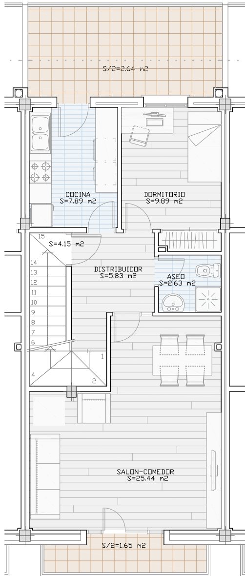
VIVIENDA 9 PLANTA PRIMERA
