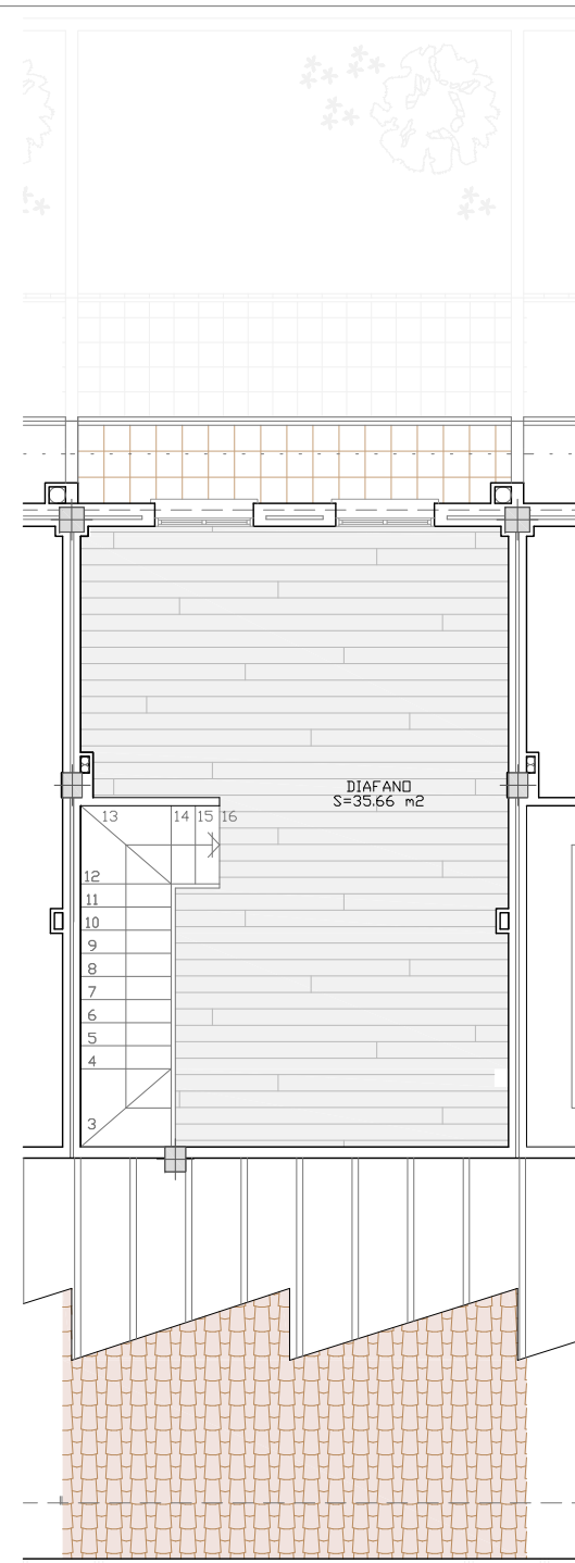
VIVIENDA 9 PLANTA BAJO CUBIERTA
